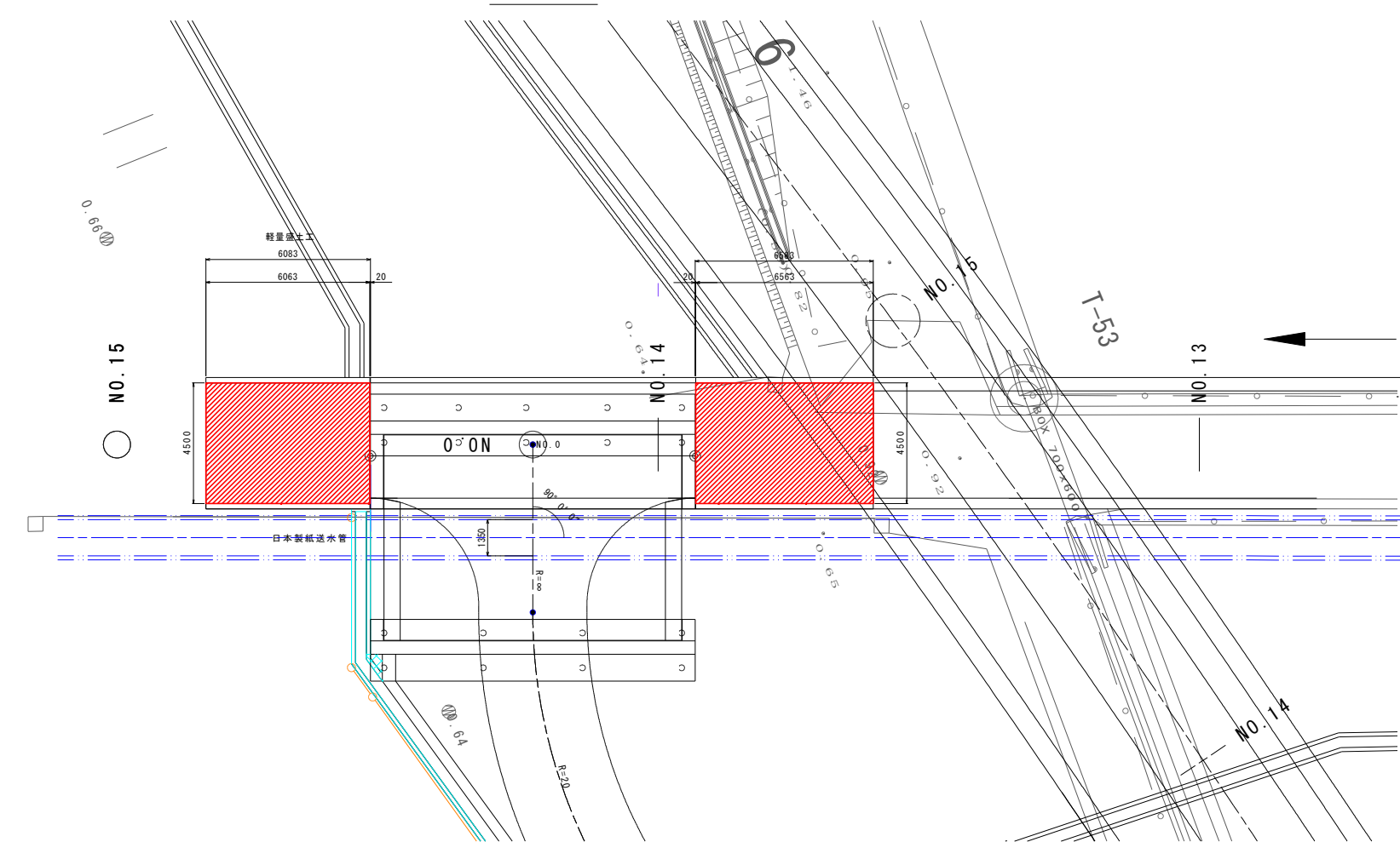
平面図
