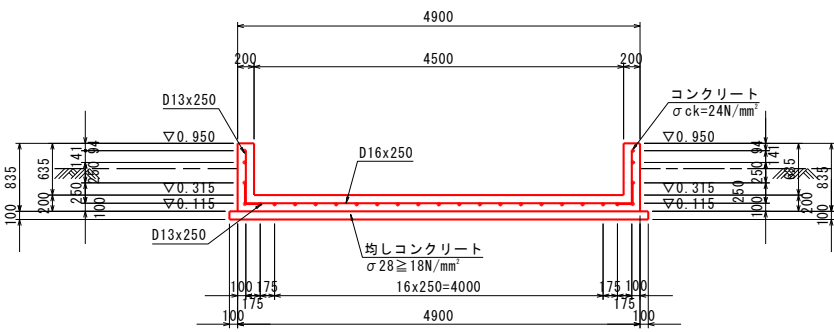
2-2断面
