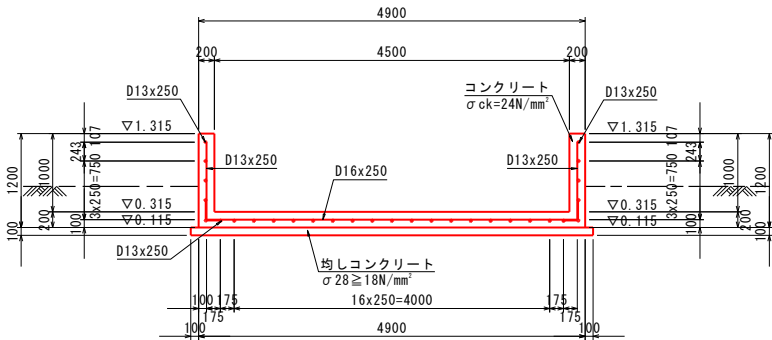
2-2断面
