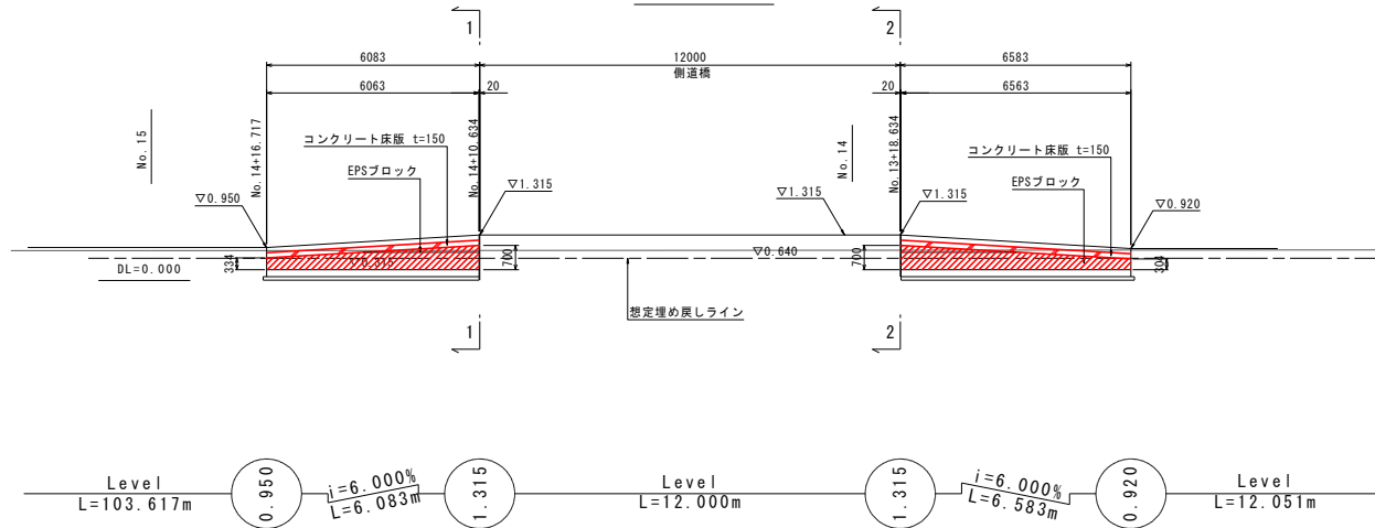
側面図
