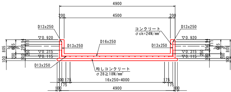
1-1断面
